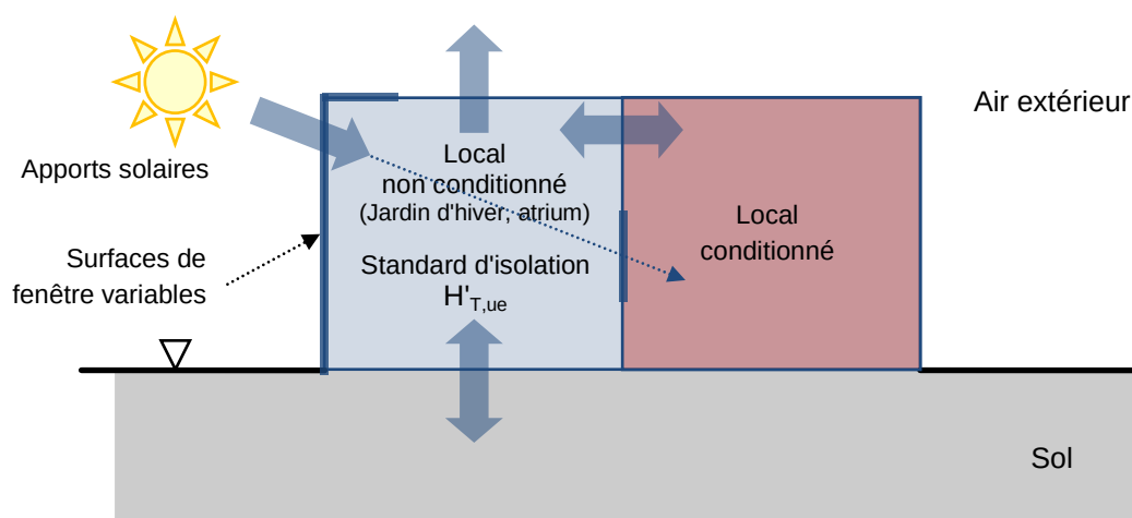
Figure 6: Schéma du modèle permettant d'analyser l'impact des zones non conditionnées exposées aux rayonnements solaires sur le bilan énergétique thermique
