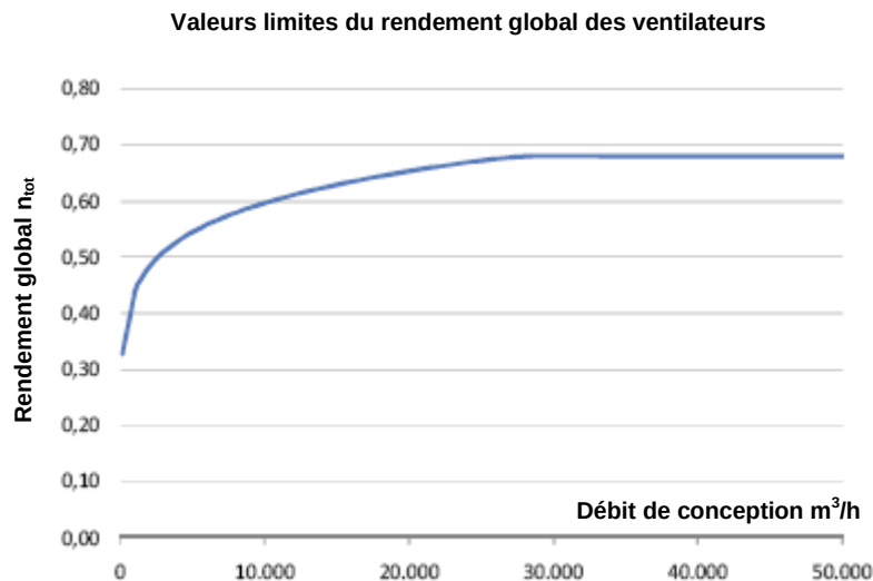
Figure 2: Valeurs limites du rendement global des ventilateurs
