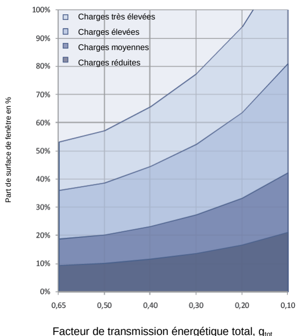
Figure 7: Estimation du niveau des apports solaires d'une zone non conditionnée en fonction de la protection solaire et de la part de surface de fenêtre respectivement de la surface de fenêtre rapportée à la surface de plancher nette.
